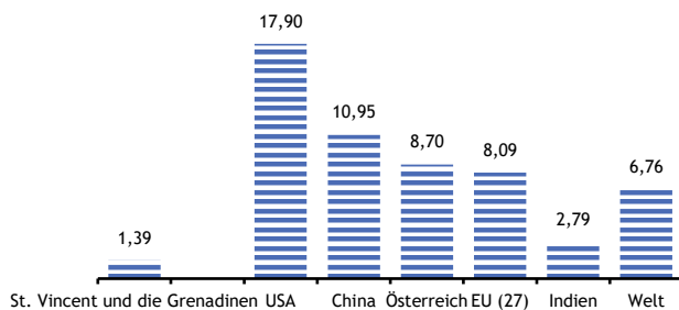
Treibhausgasemissionen 2022 in Tonnen je Einwohner
