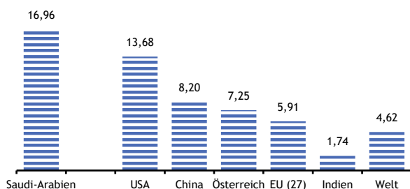
Kohlendioxidemissionen 2020 in Tonnen je Einwohner
