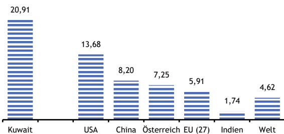
Kohlendioxidemissionen 2020 in Tonnen je Einwohner
