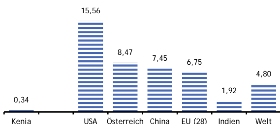
Kohlendioxidemissionen 2016 in Tonnen je Einwohner
