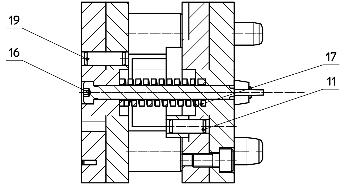
Schnitt B-B
