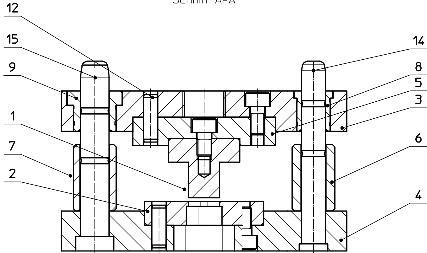
Schnitt A-A
