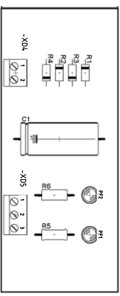
Aufbau Platine
