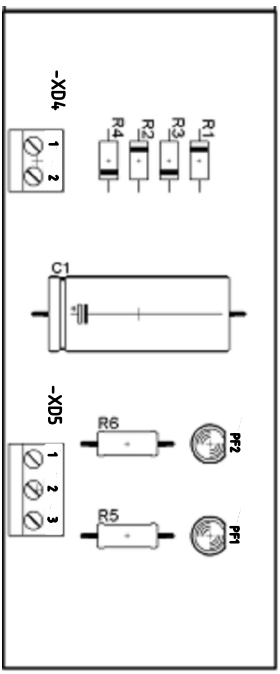
Aufbau Platine
