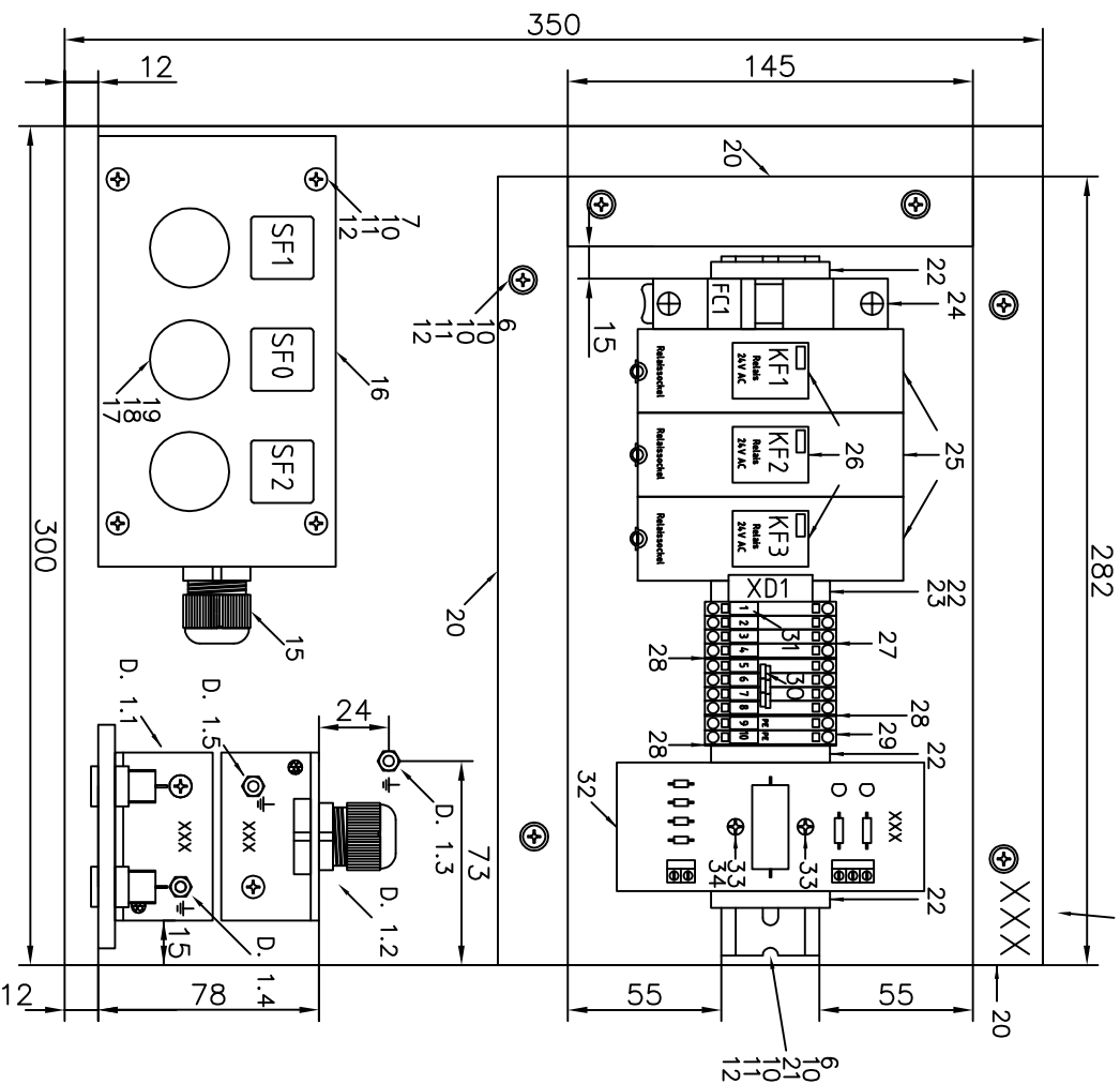
1.1 Detailzeichnung – Anschlussplatte:
