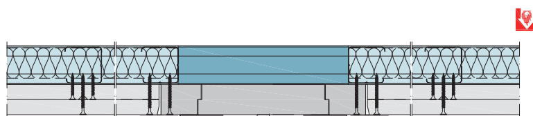
Bild 4: Einbau von Revisionsklappen
