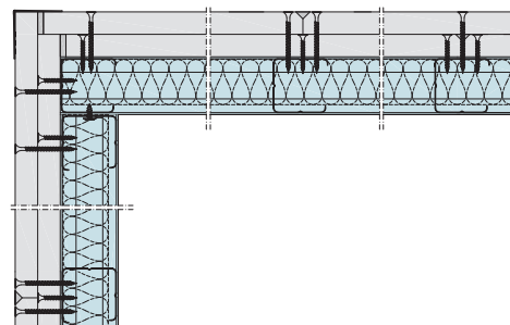
Bild 16: Eckausbildung Schachtwand
