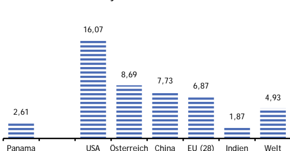
Kohlendioxidemissionen 2015 in Tonnen je Einwohner
