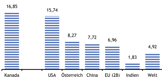
Kohlendioxidemissionen 2017 in Tonnen je Einwohner
