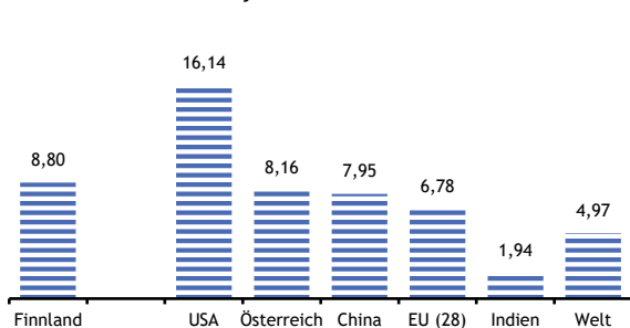
Kohlendioxidemissionen 2018 in Tonnen je Einwohner
